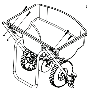
Enlevez les boulons et les écrous
