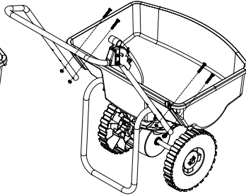
Gire la manija hacia arriba y vuelva a colocar los tornillos y las tuercas.
