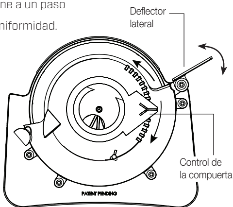
FIGURE C (Ubicación de la compuerta)
