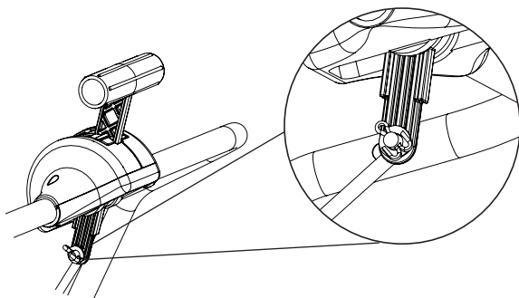
Ensamblaje Completo
